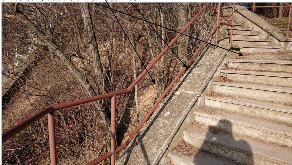
Obr.č.56 Podrobný bod číslo 5, 4
