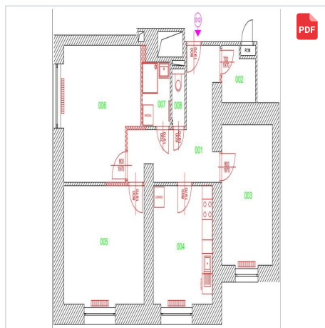
Tuckova 40 byt 12_novy stav.pdf
