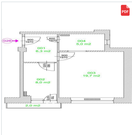
Krenova 55_byt 26_stavajici stav.pdf
